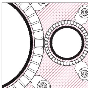
Paigaldatud kinnitusklaambrid
