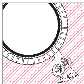
Keeratavad kinnitusklaambrid
